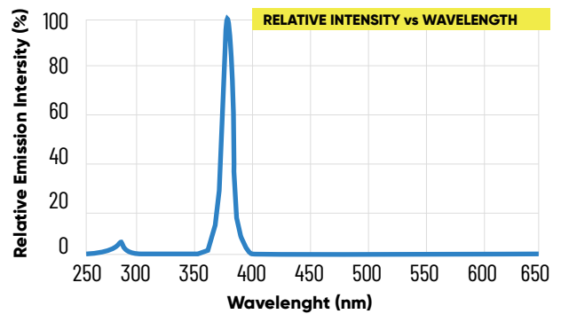
Gráfico del espectro SQD (barra UV de 30 W)
